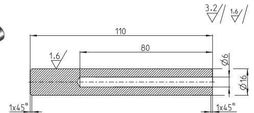
MANURHIN K'MX 632
